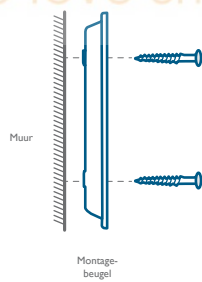
Zonder montagewig van 15°
