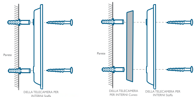
Con cuneo di montaggio a 15°
