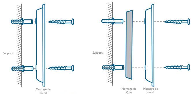
Sans cale de montage 15°
