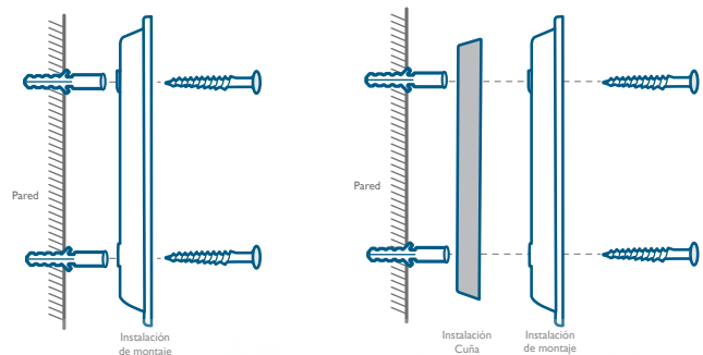
Sin cuña de montaje de 15°
