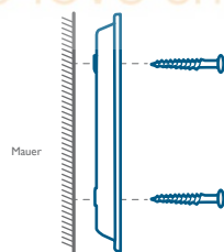
Ohne 15°-Montagekeil
