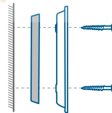
Mit 15°-Montagekeil
