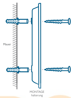
Ohne 15°-Montagekeil
